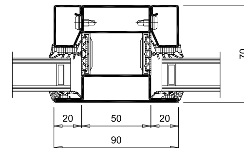
Montant - traverse
