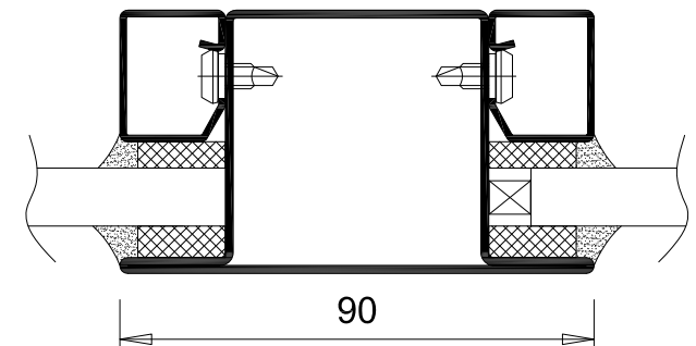
Montant - traverse
